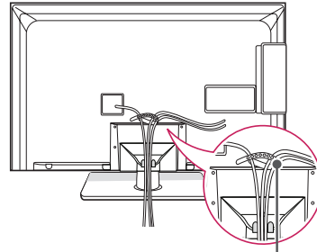
Sujetacables
