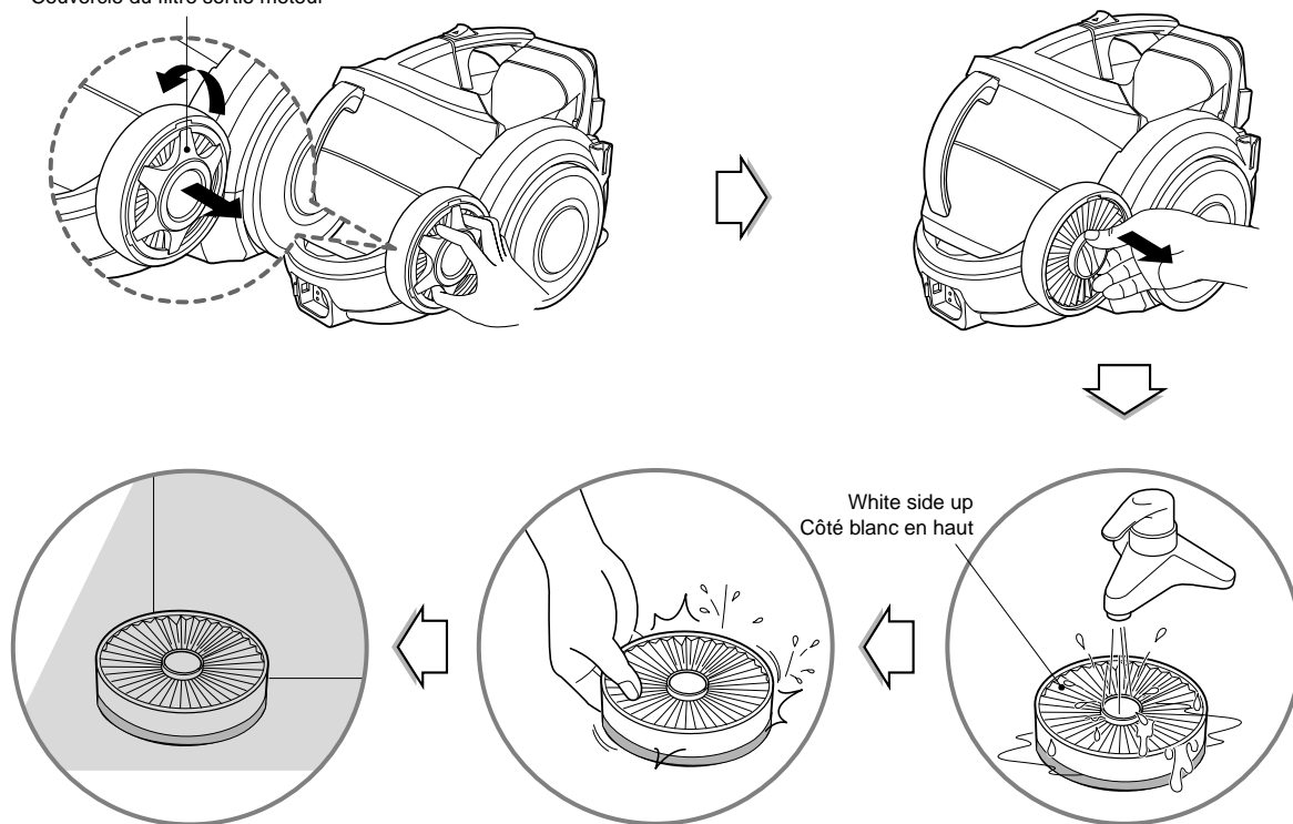
Exhaust filter cover Couvercle du filtre sortie moteur
