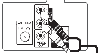
Заден панел на устройството
