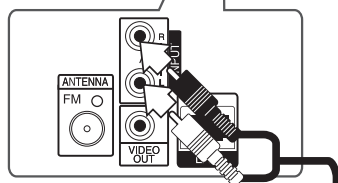
Tył urządzenia
