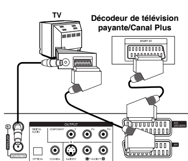
Panneau arrière du graveur
