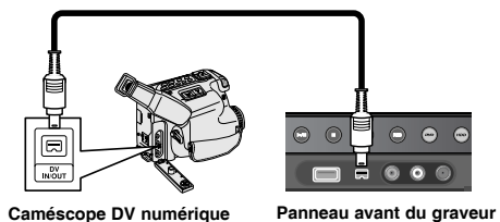
Caméscope DV numérique
