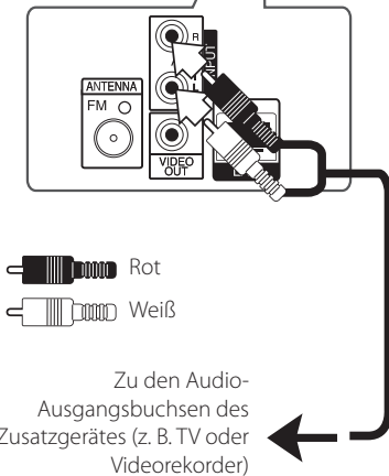
Geräterückseite
