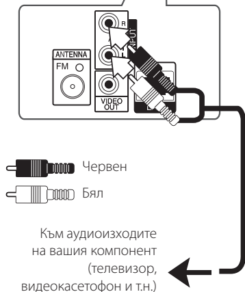
Заден панел на устройството
