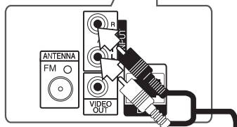
Tył urządzenia
