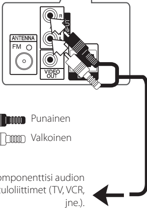
Yksikön takaosa
