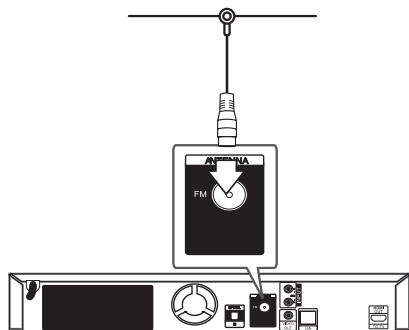
Tył urządzenia
