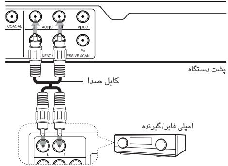
پشت دستگاه
