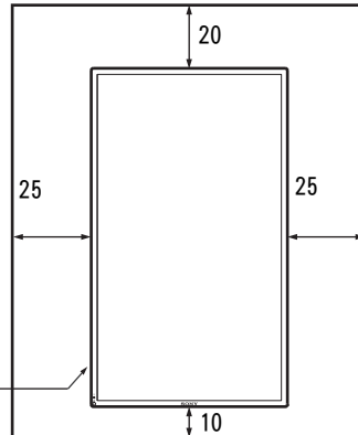
前视图
