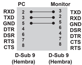
Configuraciones de 3 cables (no estándar)
