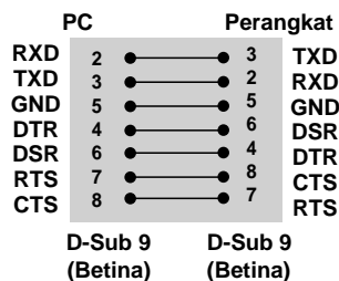
Konfigurasi 7-Kabel (Kabel RS-232C standar)
