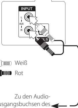
Geräterückseite
