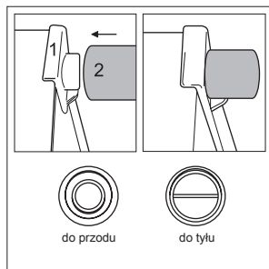
Rys. 1. Instalacja ograniczników
