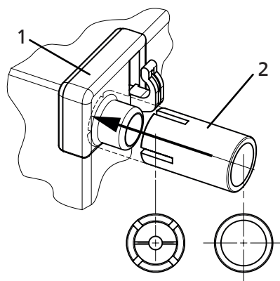
Rys. 1. Nałóż tuleje (2) na narożnik (1) i dociśnij do końca.
