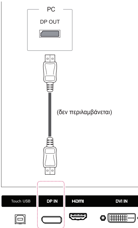
Πίσω μέρος συσκευής.
