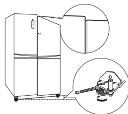
3 校平和冰箱门对齐
