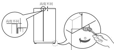
右侧高度调整螺栓
