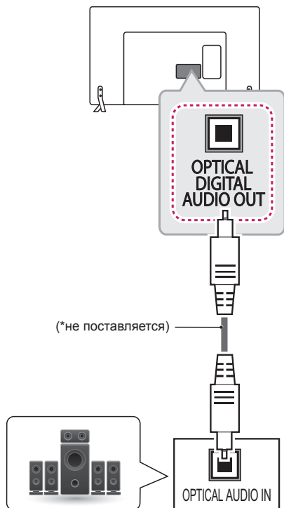
Цифровая аудиосистема
