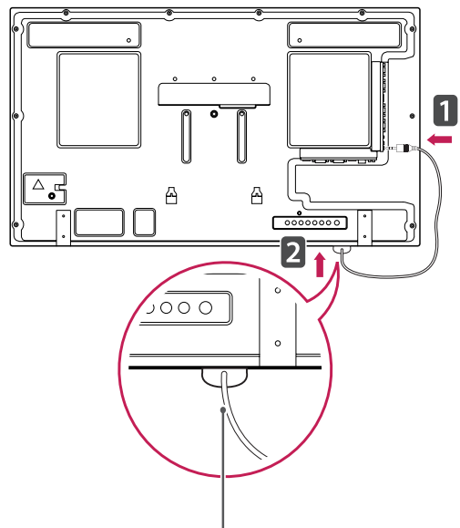
Infravörös vevőegység
