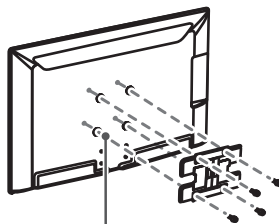
Внутрішня розпірка для настінного кронштейна
