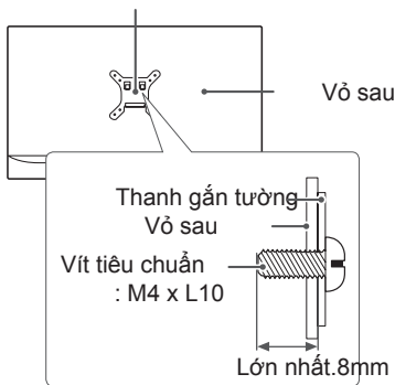
Thanh gắn tường
