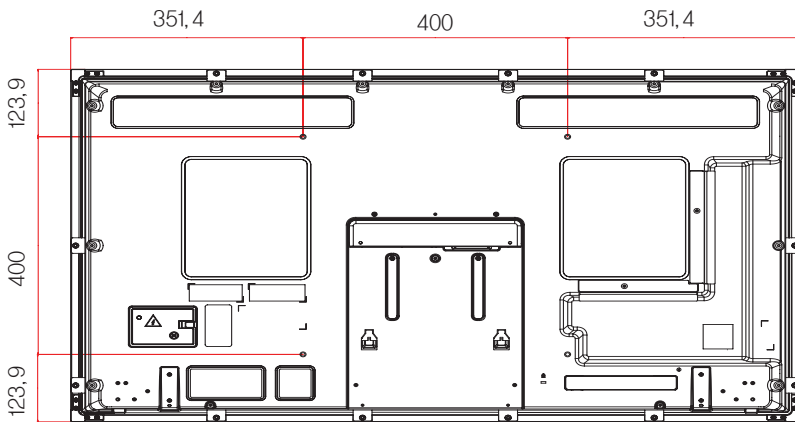
[Sekrup pemasangan di dinding] 4-M6, L10 (maks.)
