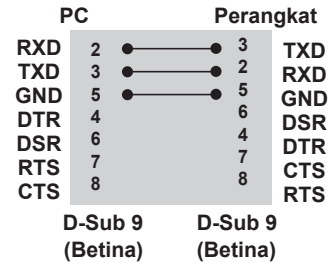
Konfigurasi 3-Kabel (Bukan Standar)
