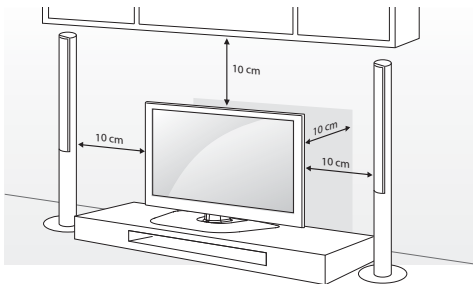
Instalação do aparelho em uma mesa.
