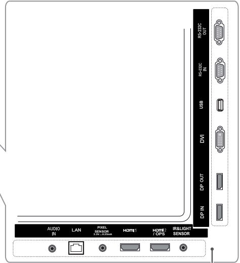
Aansluitpaneel
