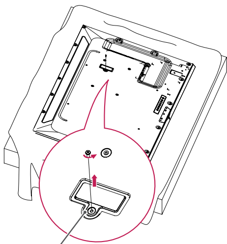
Tapa del orificio de OPS
