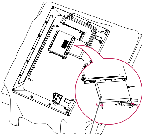
Lettore OPS
