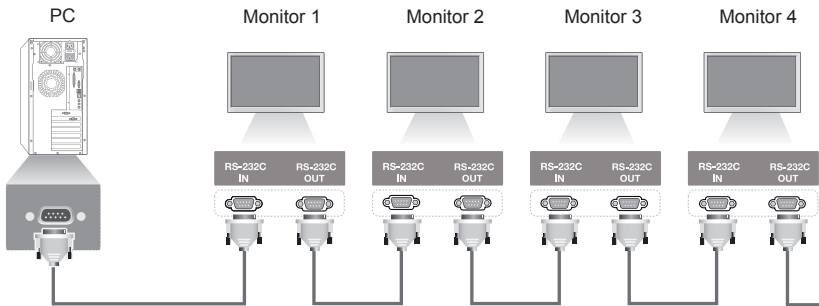
Cavo RS-232C (venduto separatamente)
