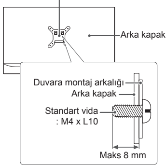
Duvara montaj arkalıği
