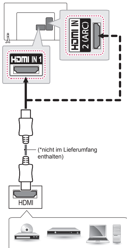
DVD / Blu-Ray / HD Kabelbox / HD STB / PC
