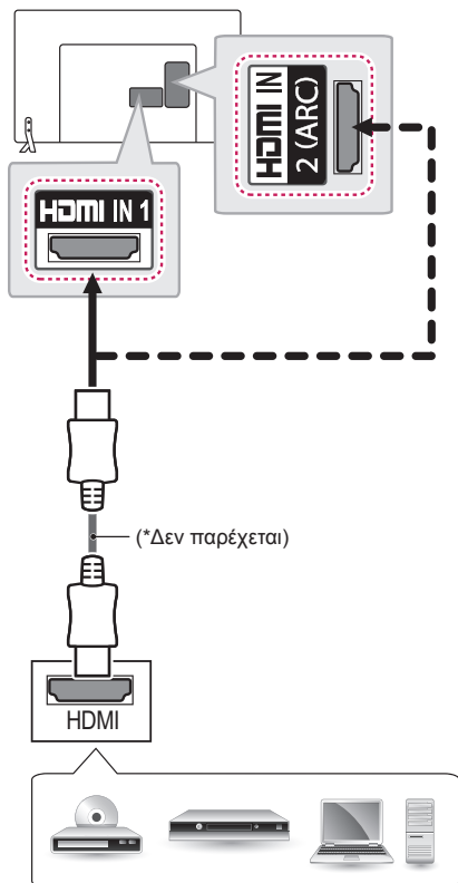
Συσκευή αναπαραγωγής DVD / Blu-Ray / HD Cable Box / HD STB / Υπολογιστή
