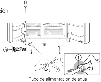
Tubo de alimentación de agua
