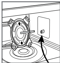
شفت موتور
