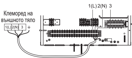
(За Сплит вътрешно тяло 5 Серия)
