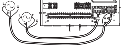
3Ø резервен нагревател (за сплит R410A вътрешно тяло 5 серия)
