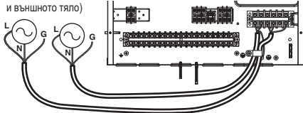
1Ø Резервен нагревател (за сплит R410A вътрешно тяло 5 серия, за сплит R32 вътрешно тяло 5 серия)
