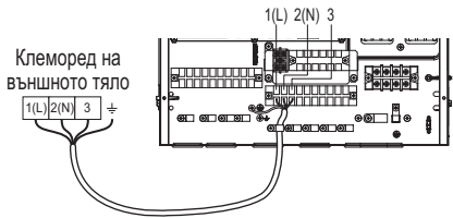
(За Сплит R410A вътрешно тяло 3 серия, за Сплит R32 вътрешно тяло 4 серия)
