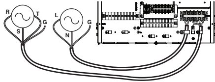
3Ø резервен нагревател (За Хидросплит)
