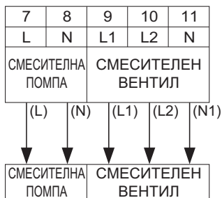
За Split вътрешно тяло 5 Серия За Hydrosplit 2-Pipe
