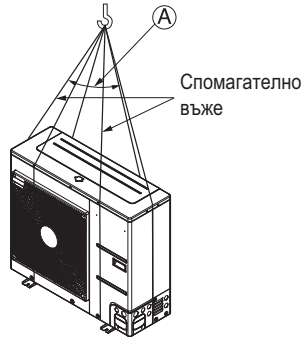
\text{\textcircled{A}} 40^\circ или по-малко
