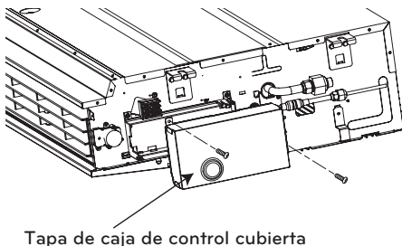
Tapa de caja de control cubierta
