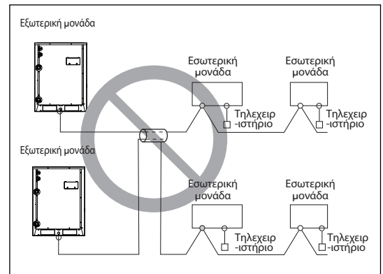
Πολυπολικό καλώδιο
