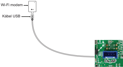
<Príklad inštalácie>
