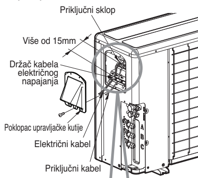
Otpušteni priključni vijak
