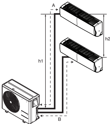
Tip višestrukih cijevi
