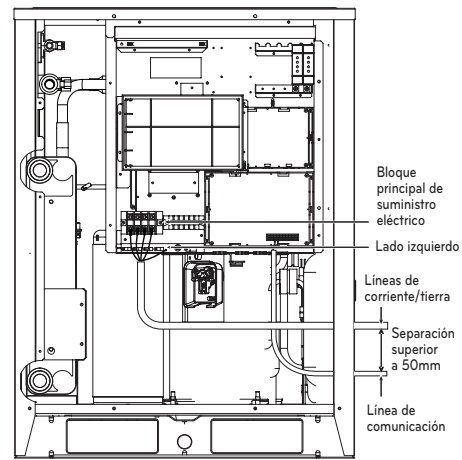
Conexión de suministro eléctrico principal
