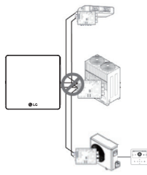
<Неправилен пример: формат на връзка RS485 STAR>
