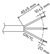
<Водач за сваляне на обвивката>
