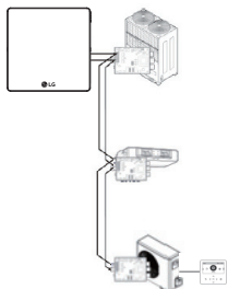
<Правилен пример: формат на връзка RS485 BUS>
