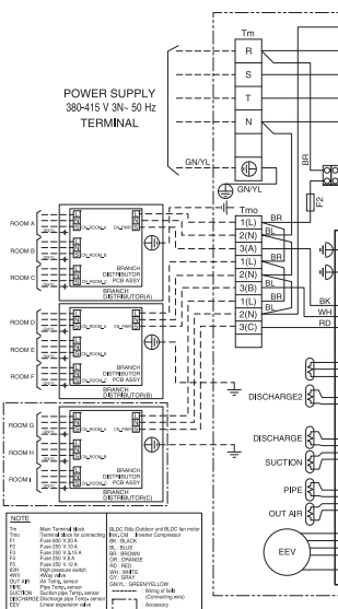
7~9 Unité (3 Ø)
