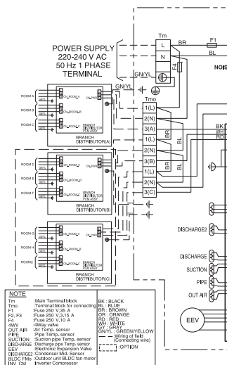
7~9 Unité (1 Ø)
