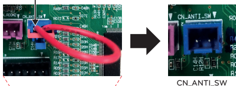
CN_ANTI_SW
