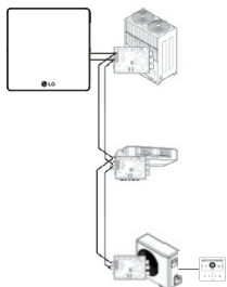
<Ispravan primer: RS485 BUS format veze>
