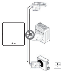
<Neispravan primer: RS485 STAR format veze>
