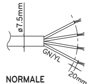
NORMALE QUERSCHNITTS-FLÄCHE 0.75mm² H07RN-F
