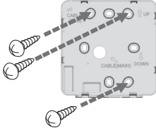
<installation d'une boîte d'encastrement à 4 orifices>
