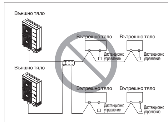
Многожилен кабел
