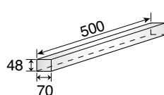
〈받침대 치수〉
