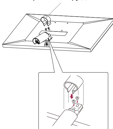
Кришка отвору для гвинтів
