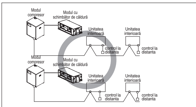
Cablu cu 2 fire ecranat
